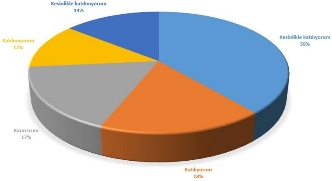
Şekil 3-Veli Paydaş Grafiği
